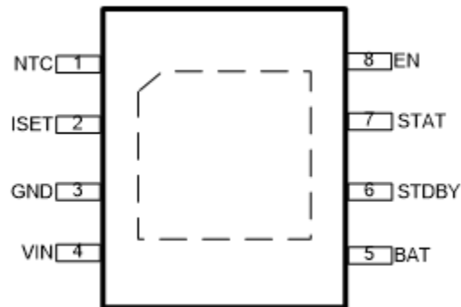
TOP VIEW(ESOP8)
