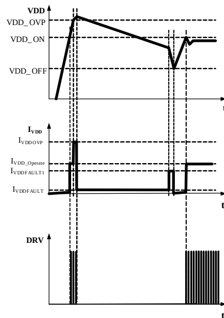
Fig. 10 VDD OVP
