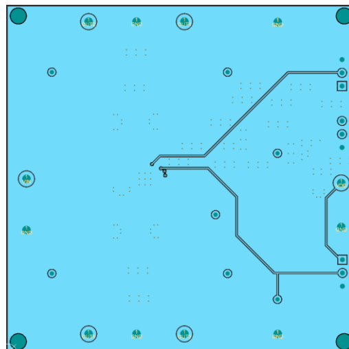
Middle Layer 2
