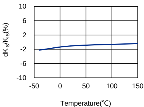
Figure 8-11. dK_{IS} / K_{IS} vs T_A ( I_L = 0.05A )
