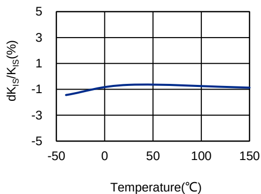
Figure 8-12. dK_{IS} / K_{IS} vs T_A ( I_L = 3A )
