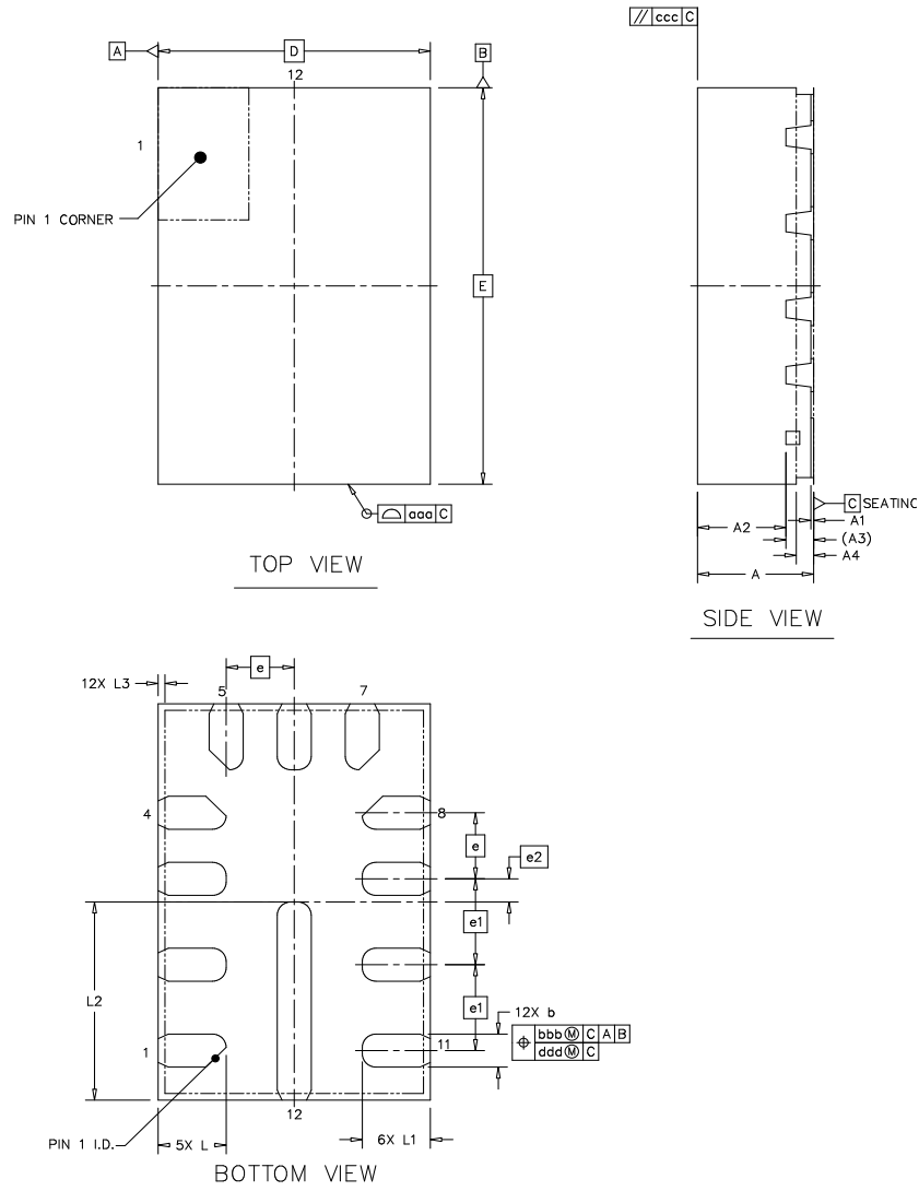
QFN-12(SC81444Q/ SC81444AQ)
