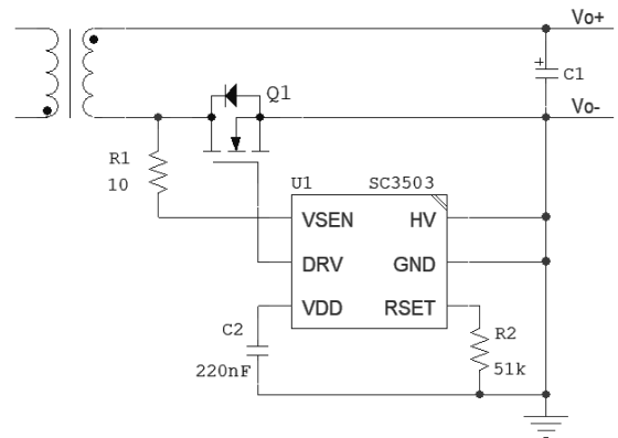
For Low V_{GS} MOSFET ( V_{DD\_REG}=6.0V )
