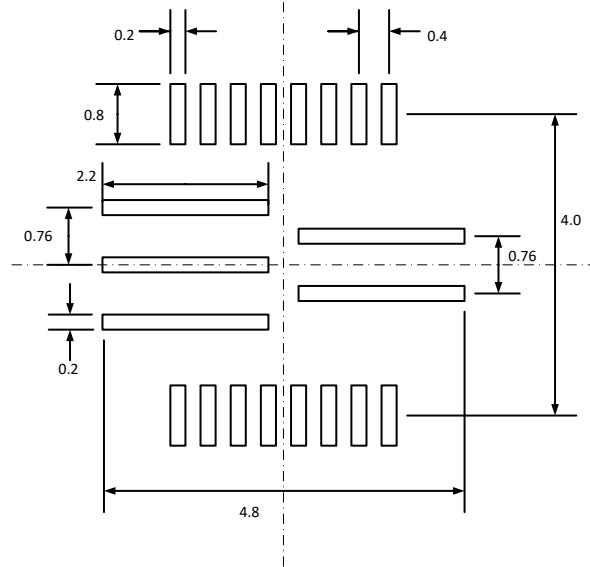
FCQFN21L (4x4x0.75)
