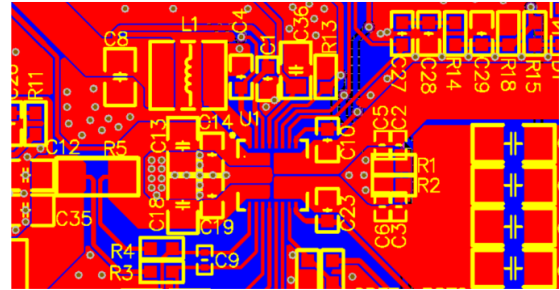
Fig6. Top Layer
