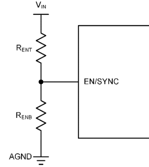
Figure 11-2. UVLO Using EN
